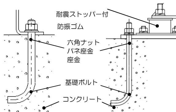
図 8. 基礎詳細図
