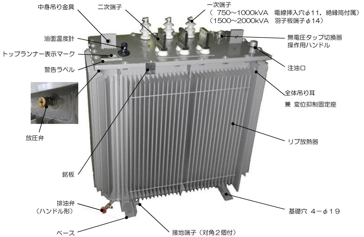
図3 空気密閉形 (三相 750~2000kVA) の各部名称
