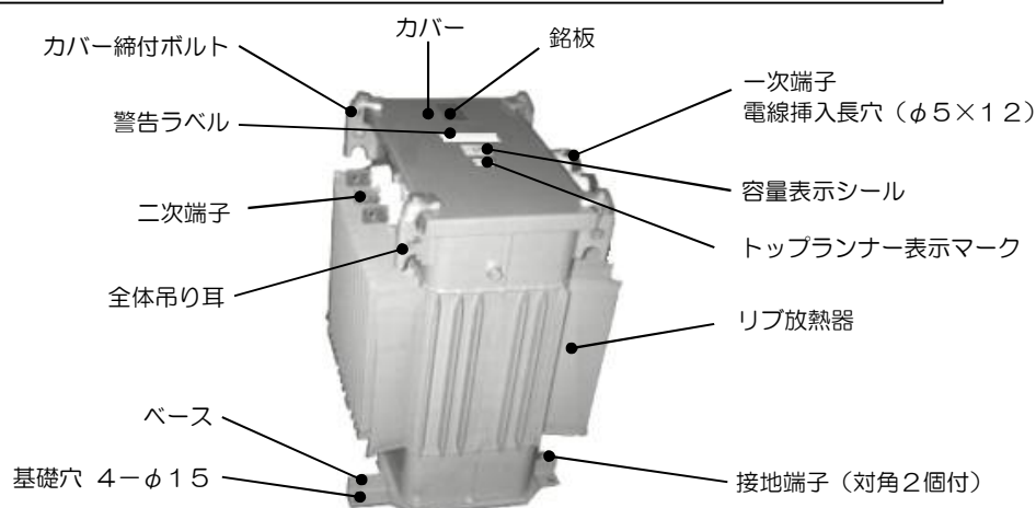
図1 空気密閉形（50kVA以下）の各部名称（単相変圧器の例）
